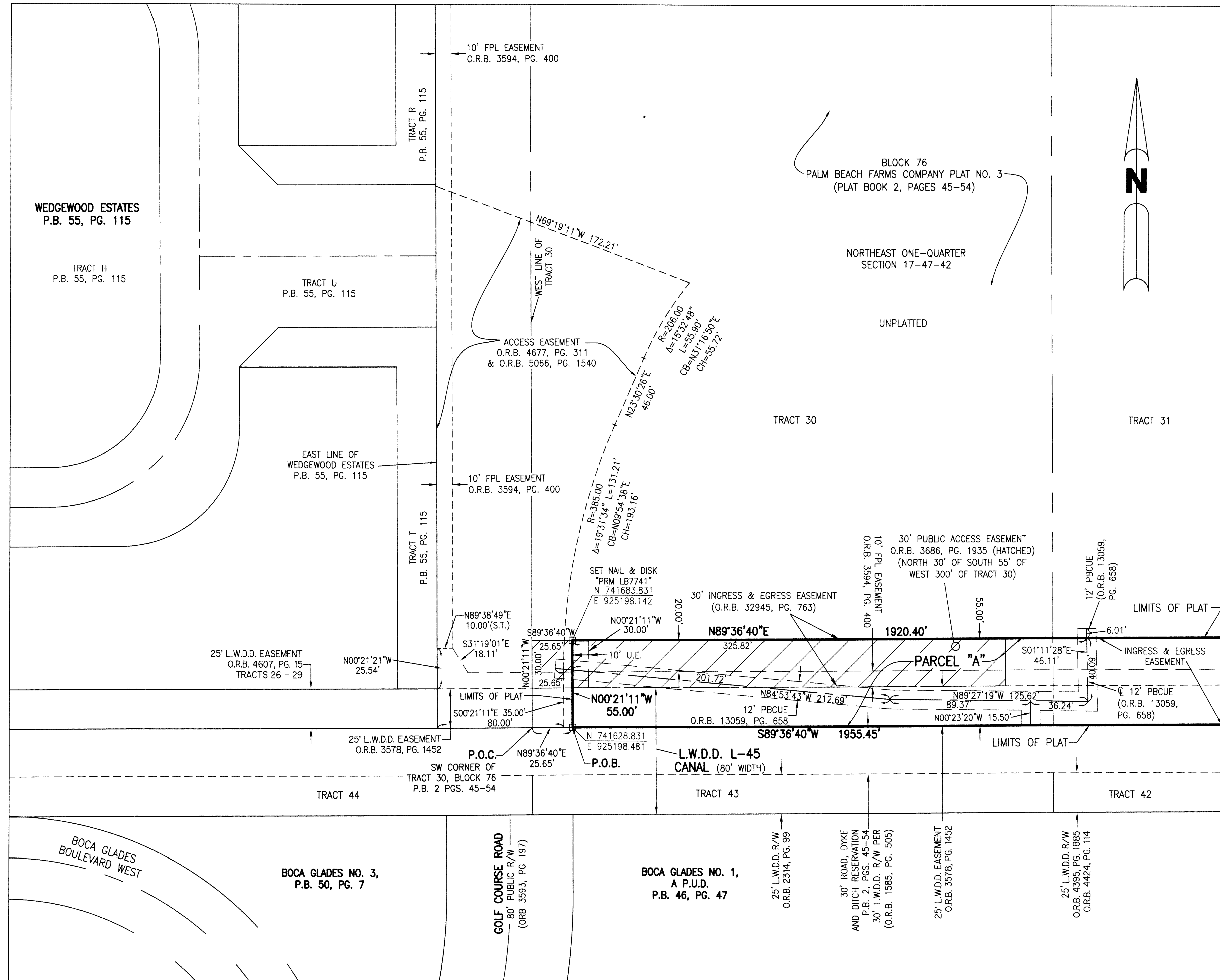
DETAIL "A" SCALE: 1"=40'
